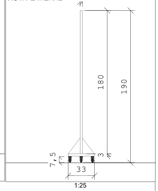
VISTA LATERAL
