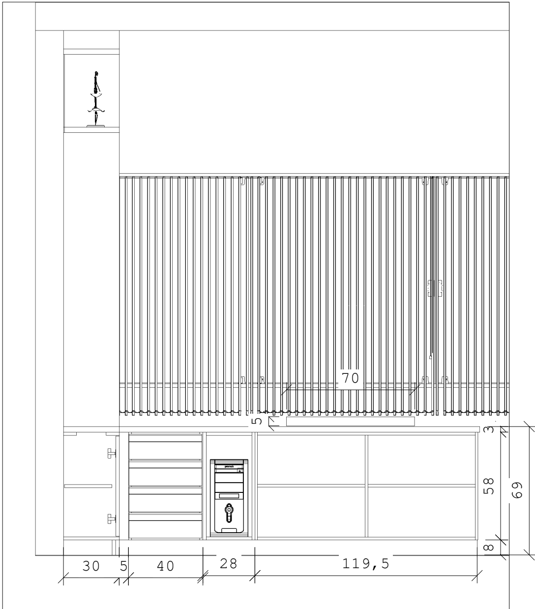
VISTA B
