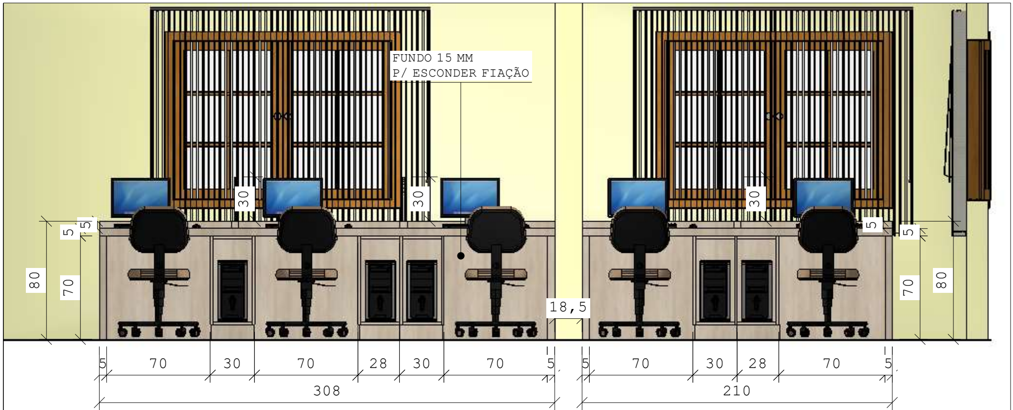
VISTA A
