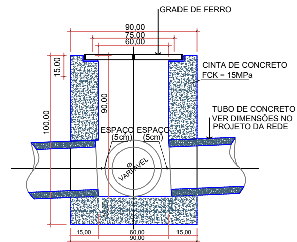
CORTE DD ESCALA: RELATIVA
