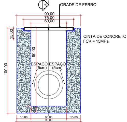
CORTE BB ESCALA: RELATIVA
