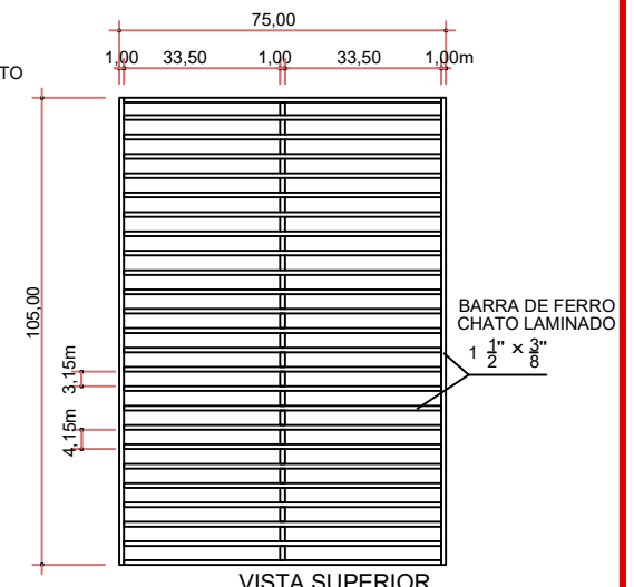
DETALHE DA GRADE SEM ESCALA DEFINIDA
