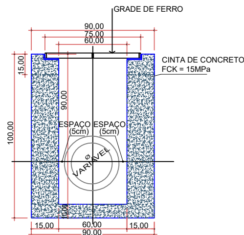
CORTE AA ESCALA: RELATIVA
