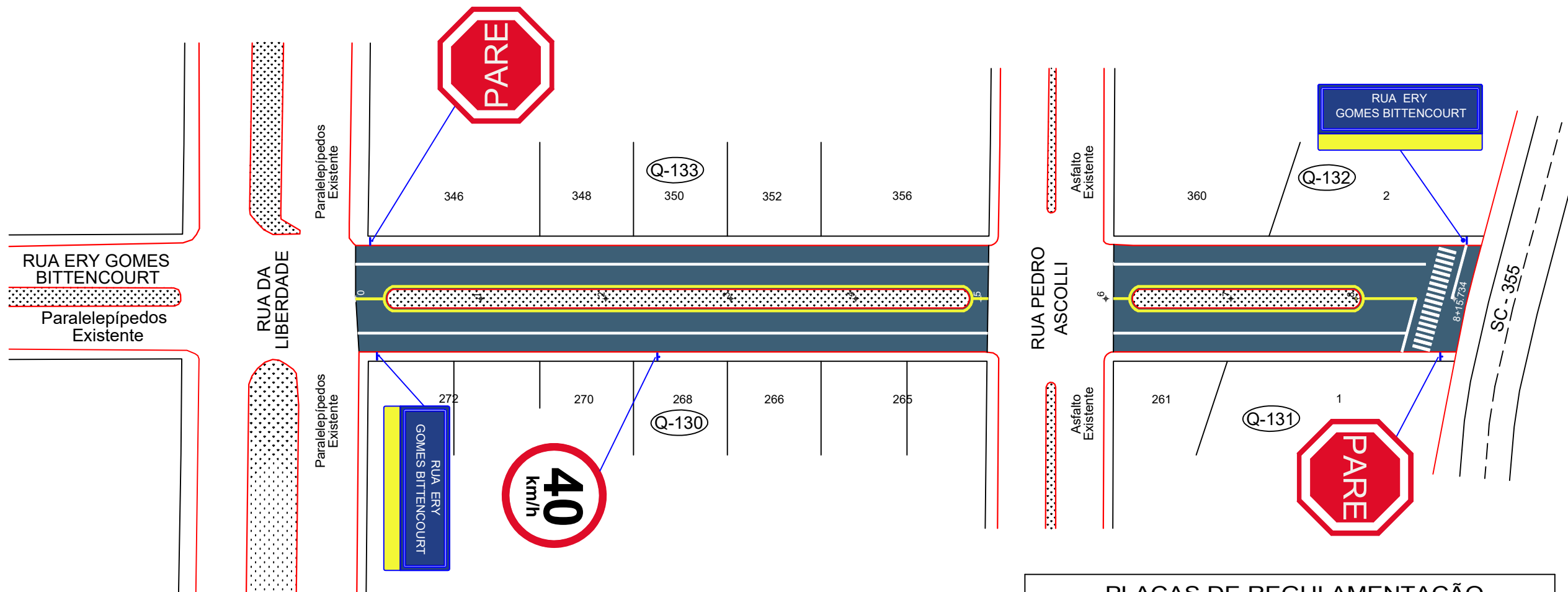
PLANTA DE SINALIZAÇÃO DA RUA ESCALA: 1/750
