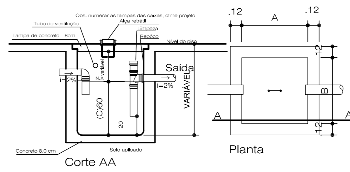
DETALHE CAIXA DE GORDURA Escala 1:25
