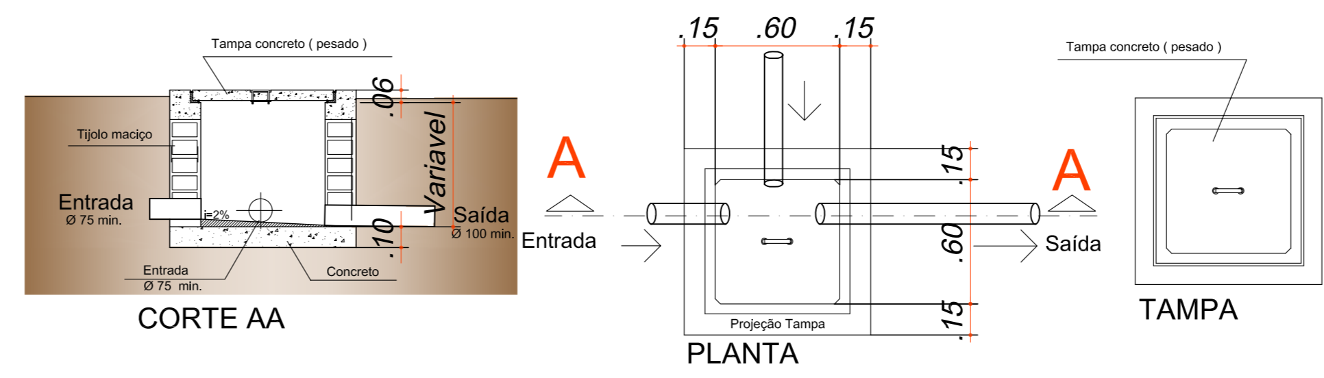
DETALHE CAIXA DE INSPEÇÃO Escala 1:25
