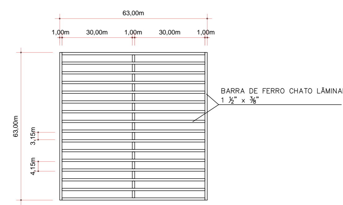
DETALHE DA GRADE Escala 1/10
