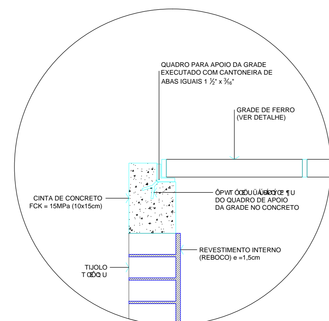
DETALHE APOIO DA GRADE Escala 1/5
