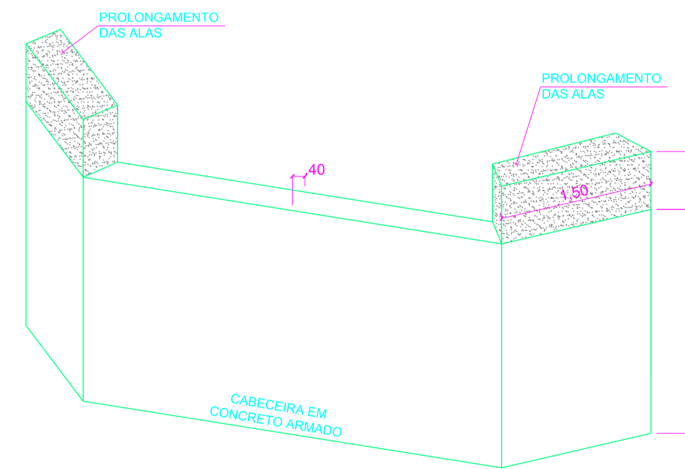
PERSPECTIVA DA CABECEIRA.....ESCALA: 1/50
