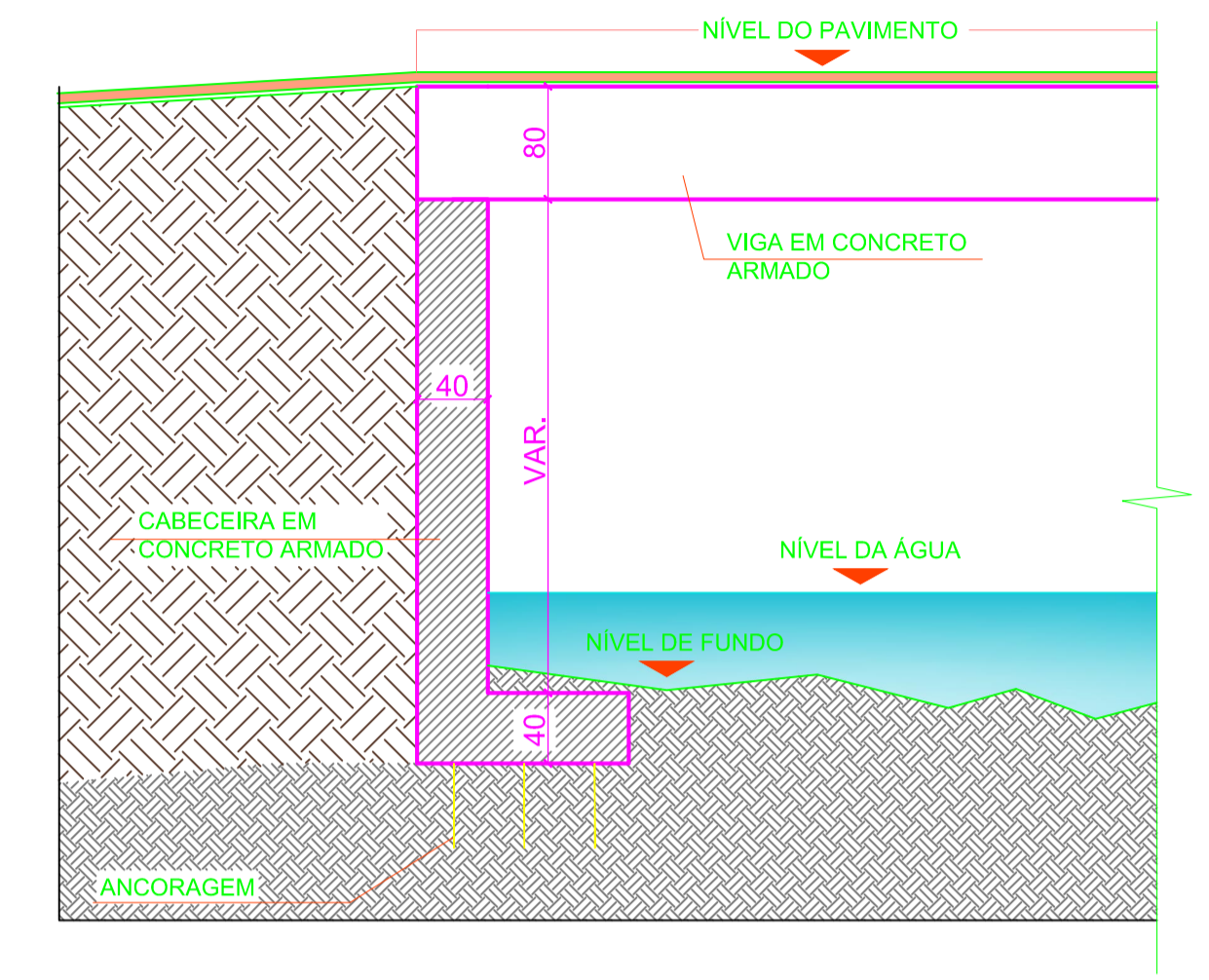
SEÇÃO LATERAL.....ESCALA: 1/50
